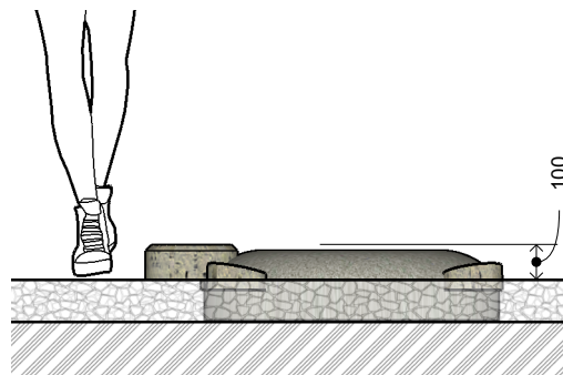
2 Front View Scale: 1:20
