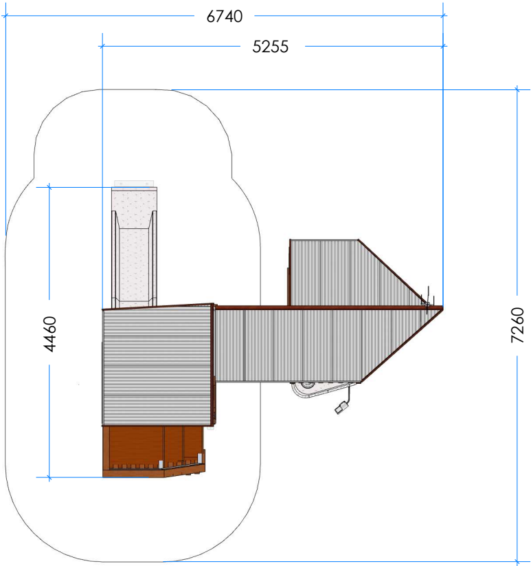
3 Top
