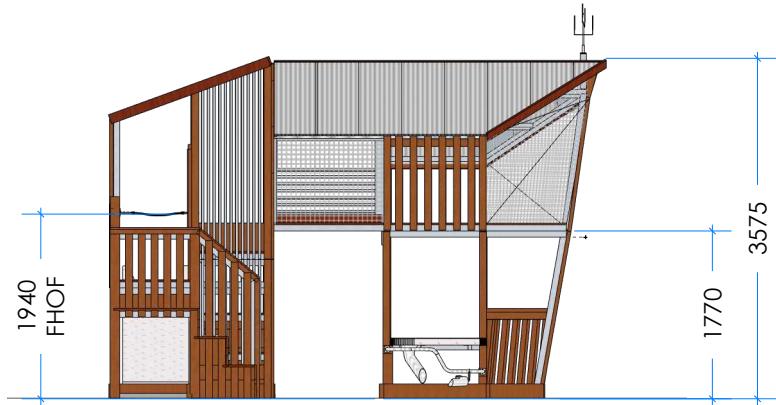
2 Elevation
