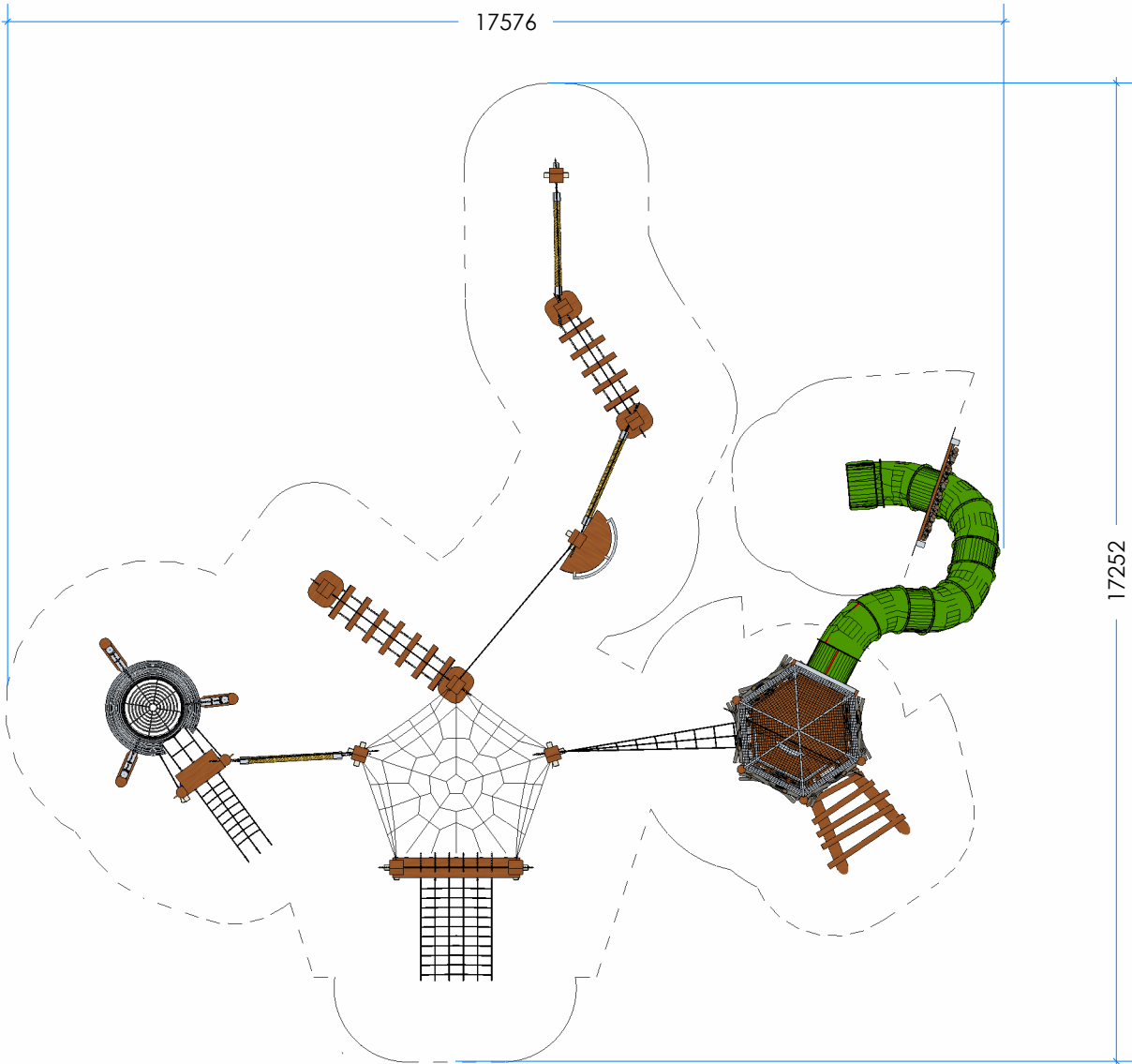
3 Top
