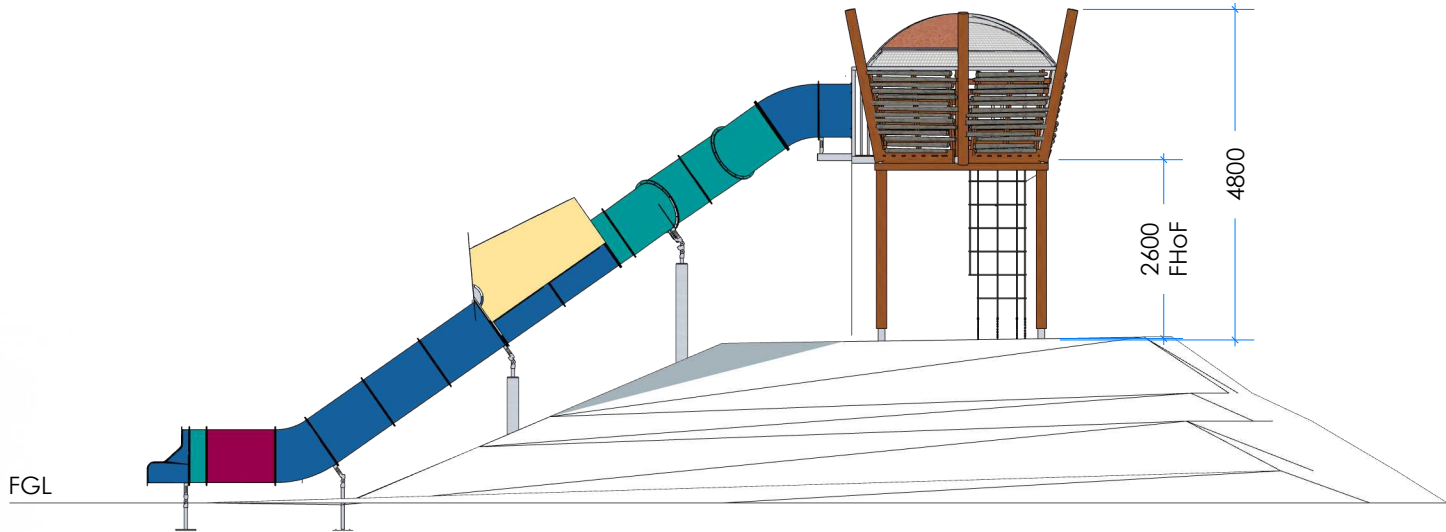
2 Elevation
