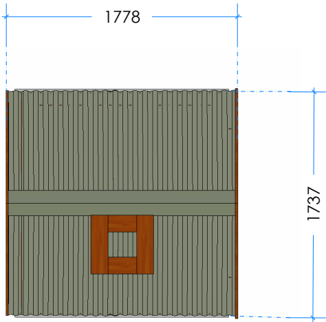
3 Top
